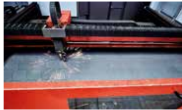
6 kW CO2 laser
